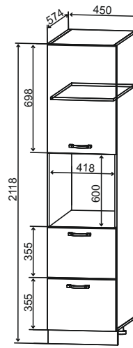
ПНЯ 450 450/2118/574 (с нишей)
