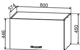
ГВПГ 800 800/450/574
