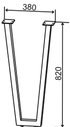
МО 550 380/820 (профиль 40x40)
