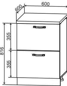
КМЯ 600 600/816/600
