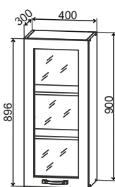
ВПС 400 400/900/300
