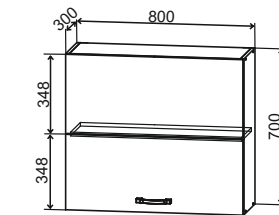
ПГПМ 800 800/700/300
