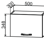
ПГ 500 500/350/300
