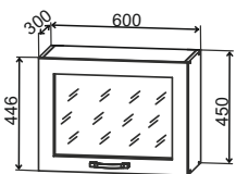
ВПГС 600 600/450/300
