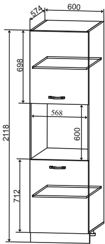
ПН 600 600/2118/574 (с нишей)
