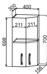
ПТ 400 400/700/300
