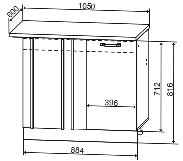
СУ 1050 1050/816/600
