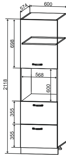
ПНЯ 600 600/2118/574 (с нишей)
