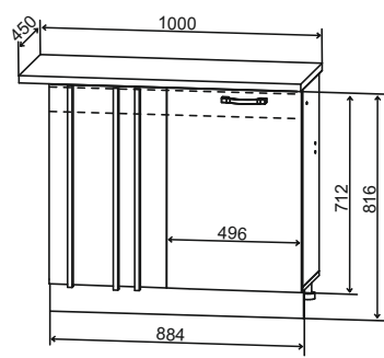
МСУ 1000 1000/816/450
