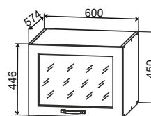
ГВПГС 600 600/450/574
