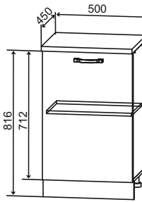
MC 500 500/816/450
