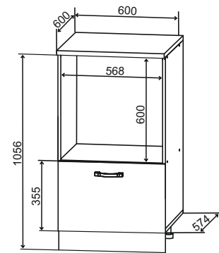
СН 600М 600/1056/600
