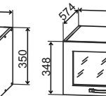
ГПГС 600 600/350/574
