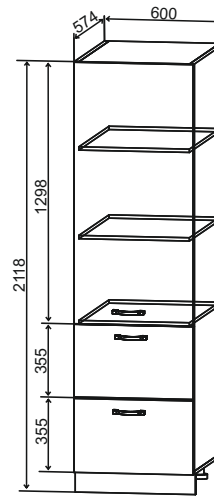
ПНЯ 600 600/2118/574
