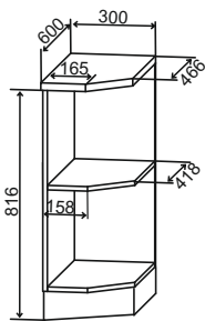
СТУ 300 300/816/600
