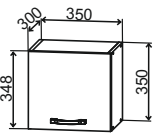
ПГ 350 350/350/300
