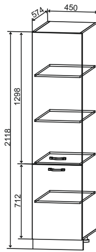
ПН 450 450/2118/574
