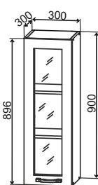
ВПС 300 300/900/300
