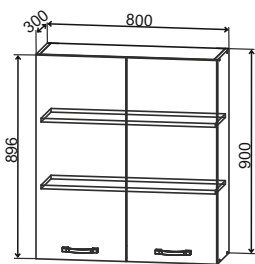
ВП 800 800/900/300
