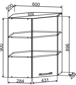
ВПУ 600 600/900/600
