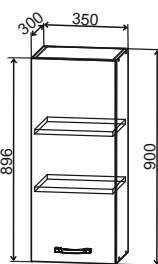
ВП 350 350/900/300
