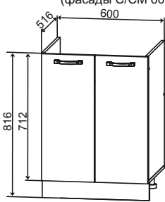
Вариант 1 (фасады С/СМ 600)
