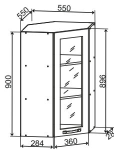
ВПУС 550 550/900/550
