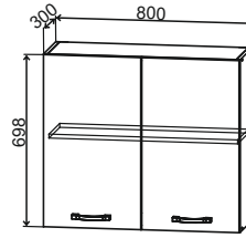
П 800 800/700/300
