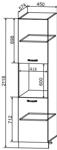
ПН 450 450/2118/574 (с нишей)
