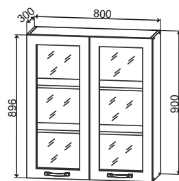
ВПС 800 800/900/300
