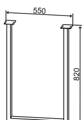
МО 495 550/820 (профиль 40x40)
