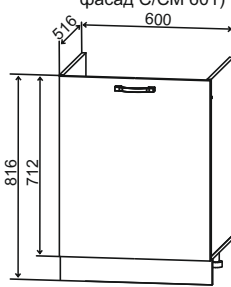
Вариант 2 фасад С/СМ 601)
