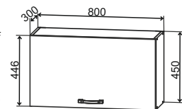
ВПГ 800 800/450/300
