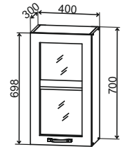
ПС 400 400/700/300
