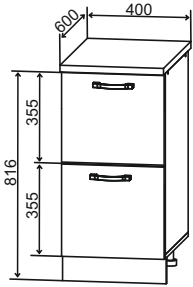
СК2 400 400/816/600
