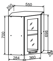
ПУС 550 550/700/550
