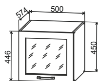
ГВПГС 500 500/450/574
