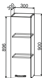
ВП 300 300/900/300
