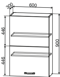
ВПГПМ 600 600/900/300
