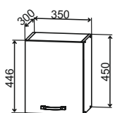
ВПГ 350 350/450/300
