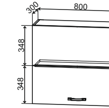
ПГПМ 800 800/700/300
