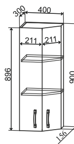
ВПТ 400 400/900/300
