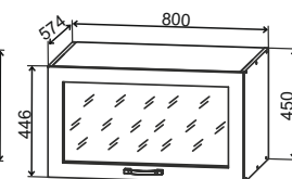
ГВПГС 800 800/450/574
