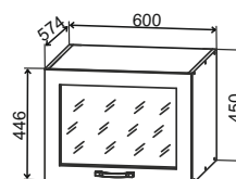
ГВПГС 600 600/450/574
