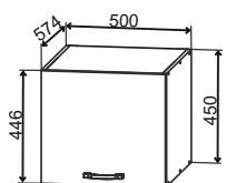
ГВПГ 500 500/450/574
