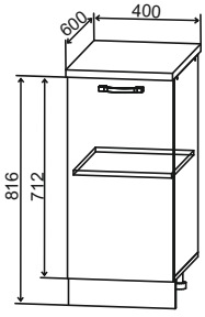
С 400 400/816/600
