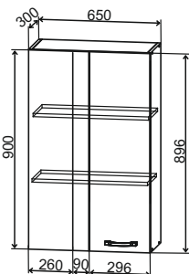
ВПУ 650 650/900/300
