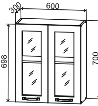
ПС 600 600/700/300
