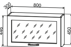
ВПГС 800 800/450/300
