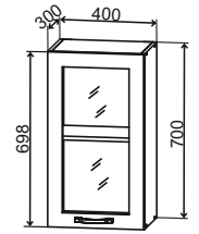
ПС 400 400/700/300
