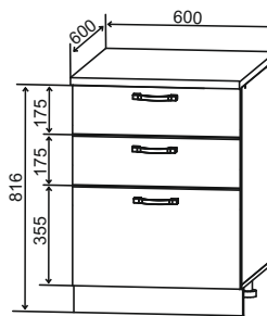
СМЯ 600 600/816/600
