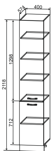
ПН 400 400/2118/574
