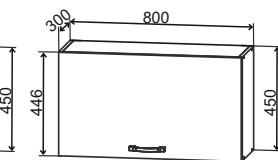
ВПГ 800 800/450/300
