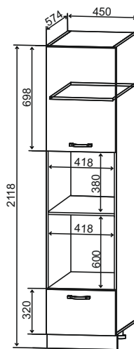
ПНС 450 450/2118/574
