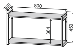
ОПМВГ 800 800/450/300 (профиль 20*20)
