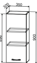
ВП 350 350/900/300
