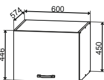
ГВПГ 600 600/450/574
