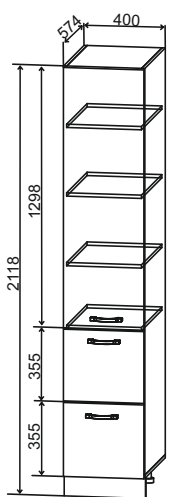
ПНЯ 400 400/2118/574
