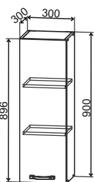
ВП 300 300/900/300
