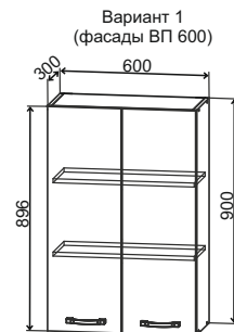
ВП 600 600/900/300
