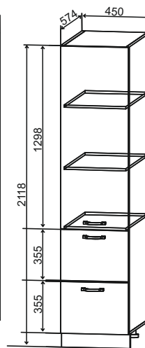
ПНЯ 450 450/2118/574
