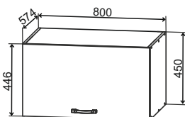
ГВПГ 800 800/450/574
