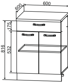
С1YШ 600 600/816/600
