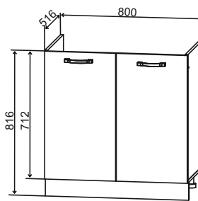
CM 800 800/816/516
