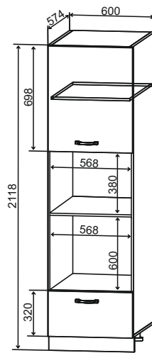
ПНС 600 600/2118/574
