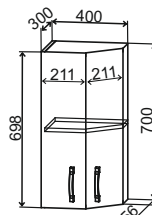
ПТ 400 400/700/300
