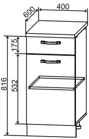
С1YШ 400 400/816/600
