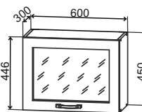
ВПГС 600 600/450/300
