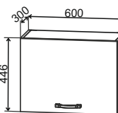
ВПГ 600 600/450/300
