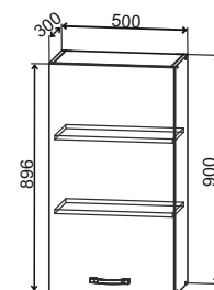
ВП 500 500/900/300
