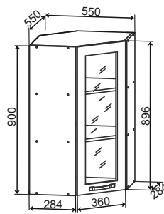
ВПУС 550 550/900/550
