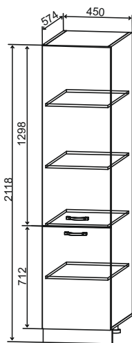
ПН 450 450/2118/574
