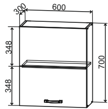
ПГПМ 600 600/700/300
