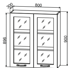
ВПС 800 800/900/300
