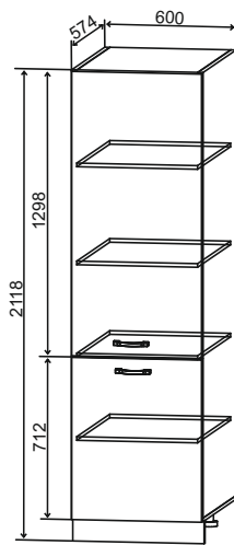
ПН 600 600/2118/574
