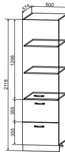
ПНЯ 600 600/2118/574
