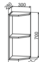
ПТУ 300 300/700/280
