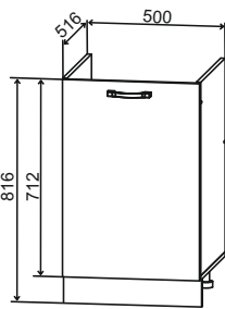
CM 500 500/816/516
