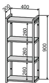
ОПМВ 400 400/900/300 (профиль 20*20)
